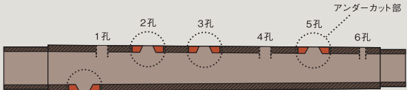
アンダーカットの形状図
