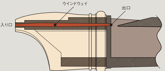
ウインドウェイの形状図
